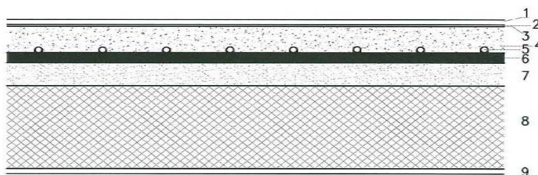
Esempio illustrato del solaio tra appartamenti
