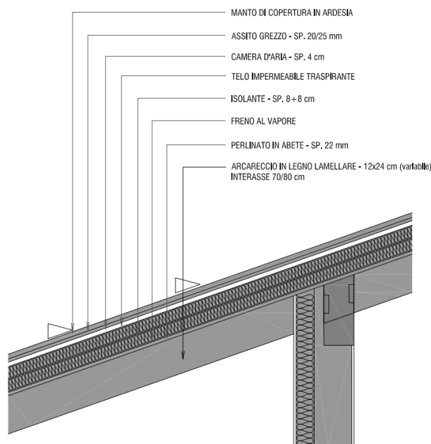
Stratigrafia pacchetto isolante tetto di copertura.
