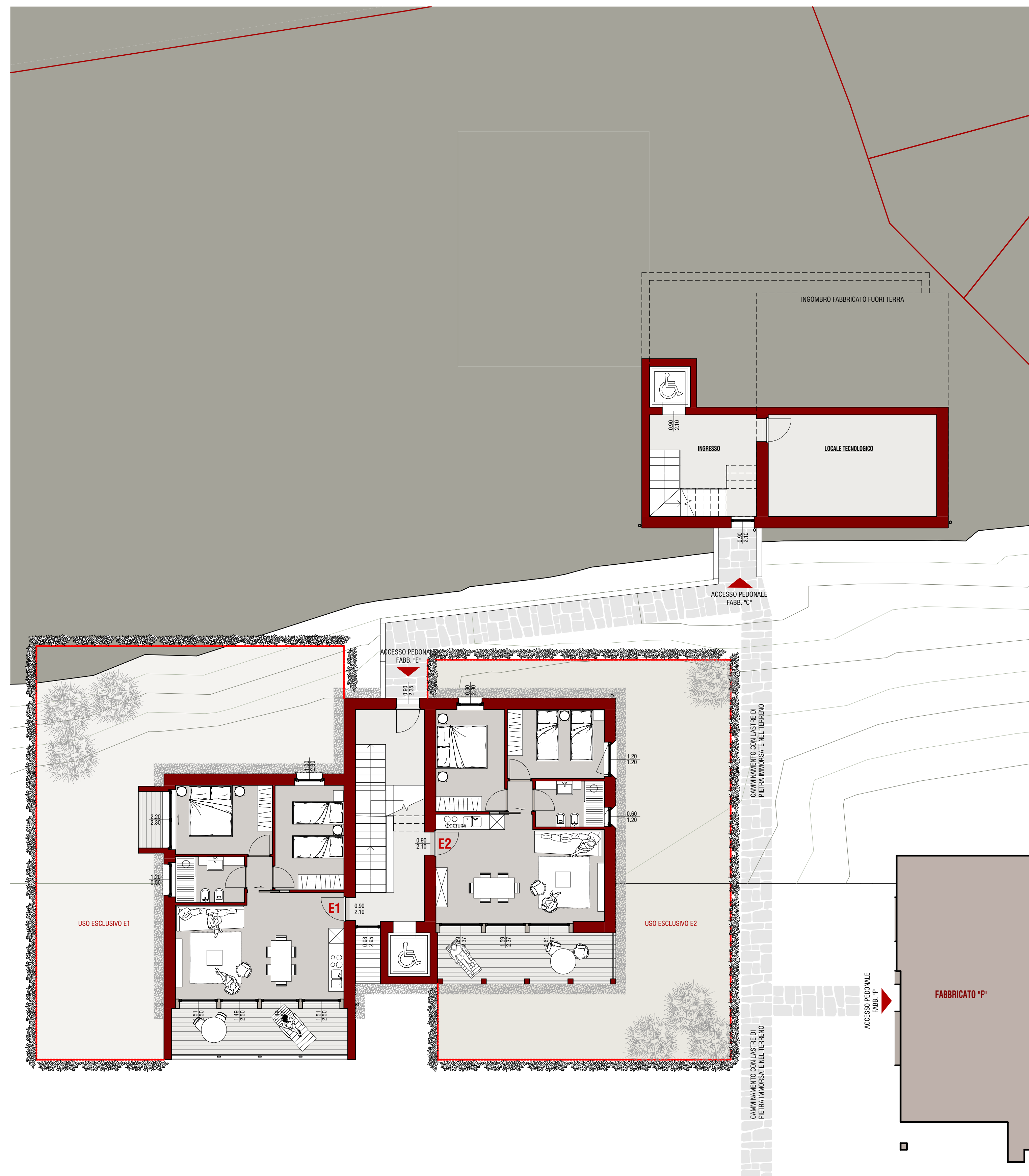
PIANO TERRA FABB. "E" - INTERRATO FABB. "C" 1 : 100
