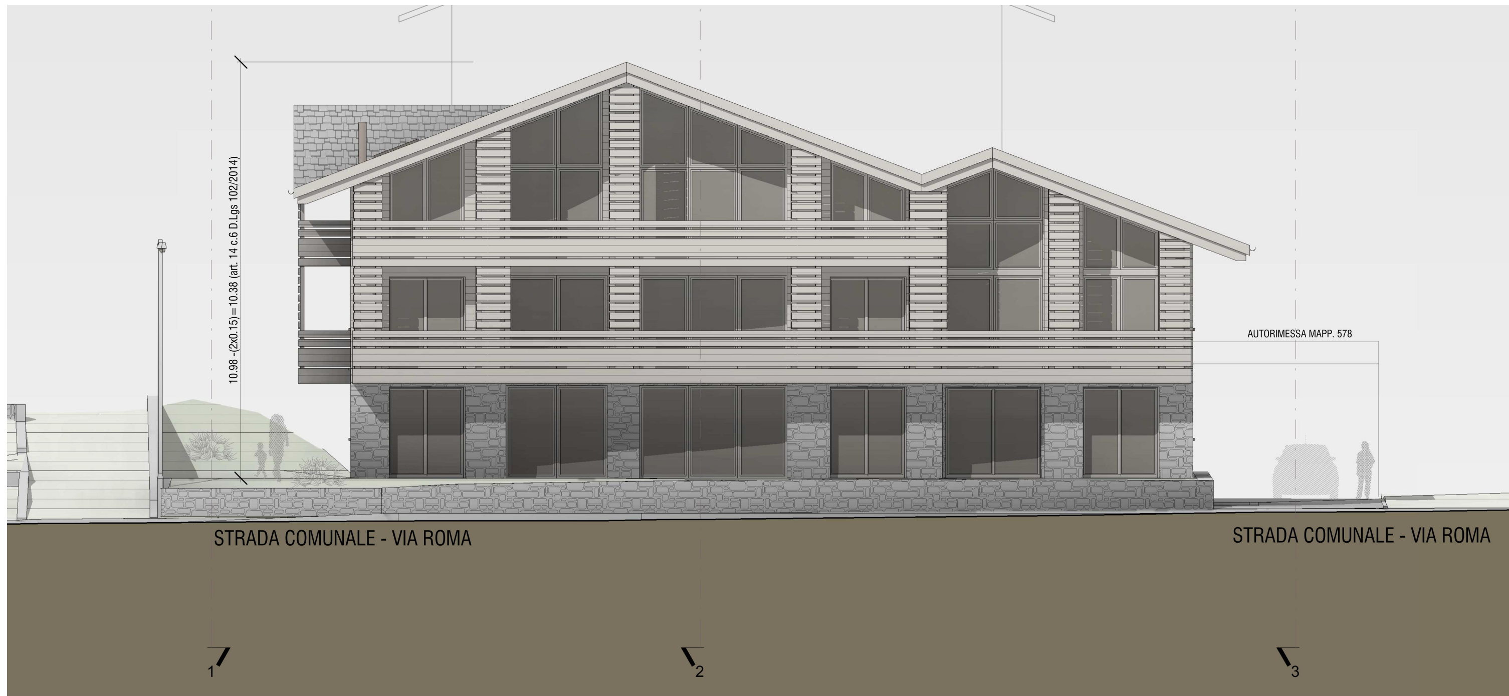
PROSPETTO EST - SEZ. 4-4
