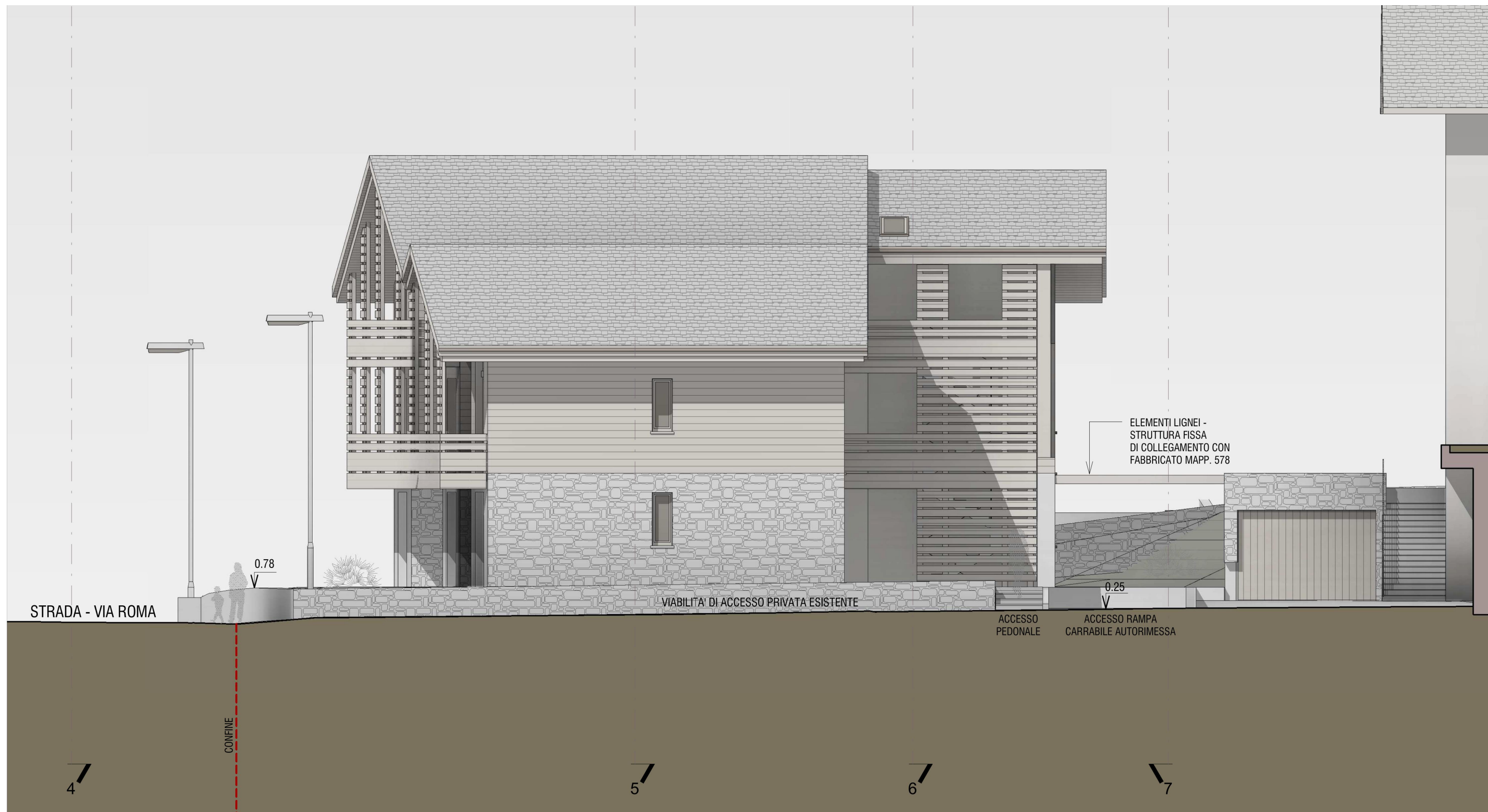
PROSPETTO NORD - SEZ. 3-3
