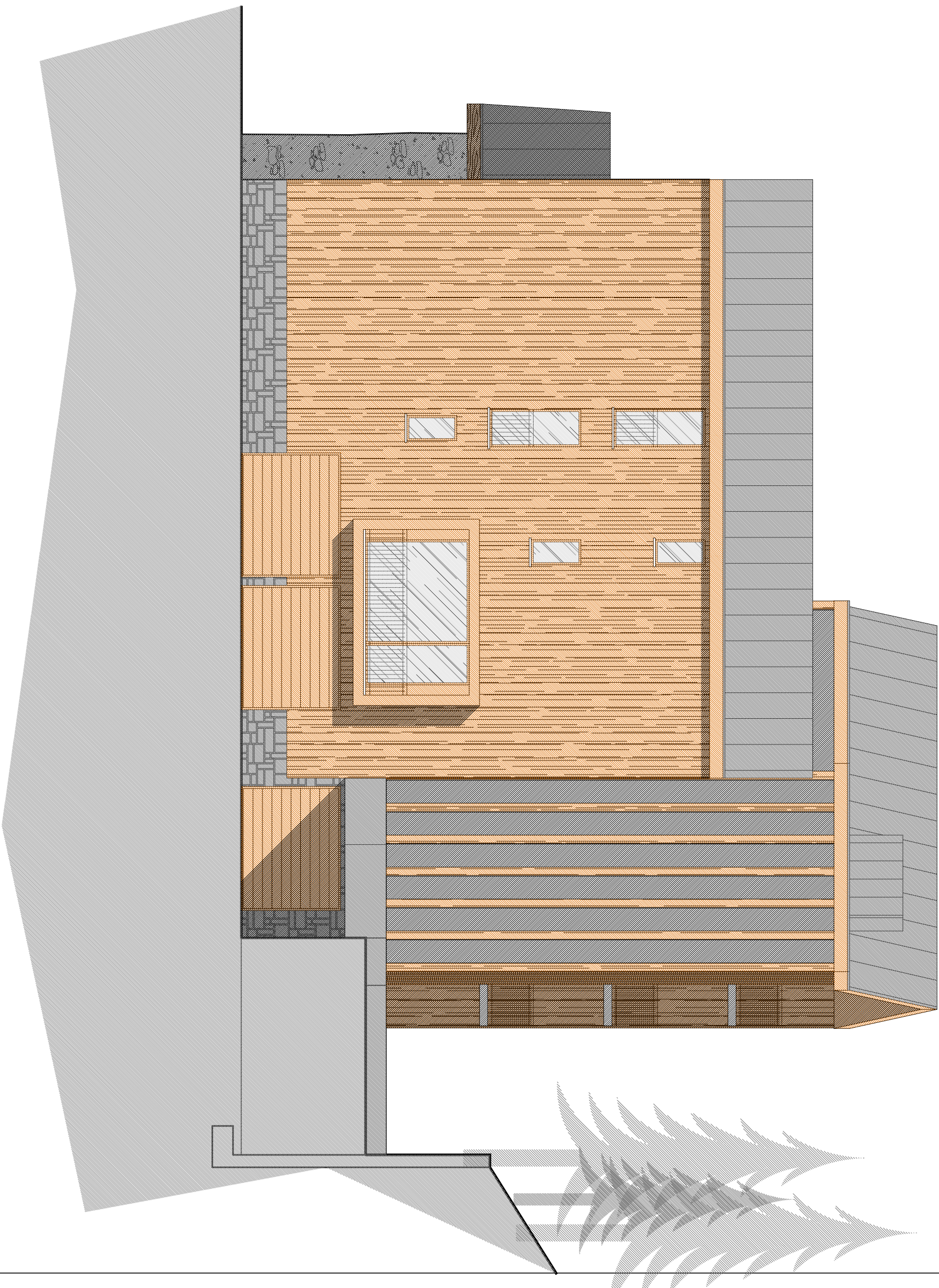
Prospetto Nord Scala 1:100
